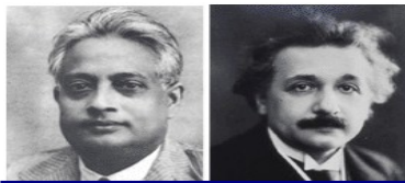
Bose - Einstein
